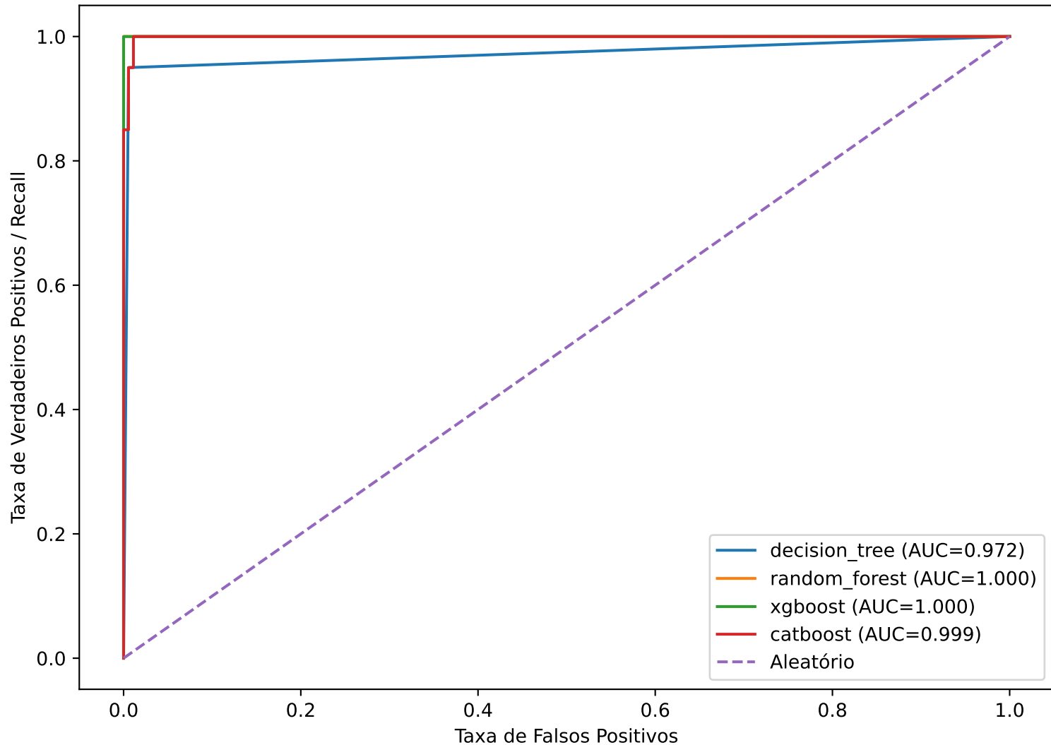
Curvas ROC — Comparação dos Modelos
